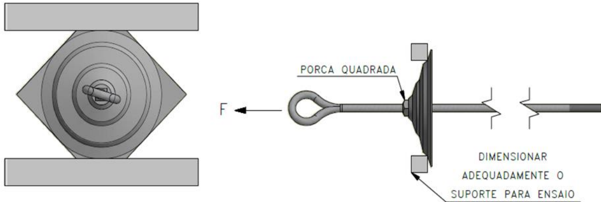
Figura 2 - Detalhe para Ensaio
