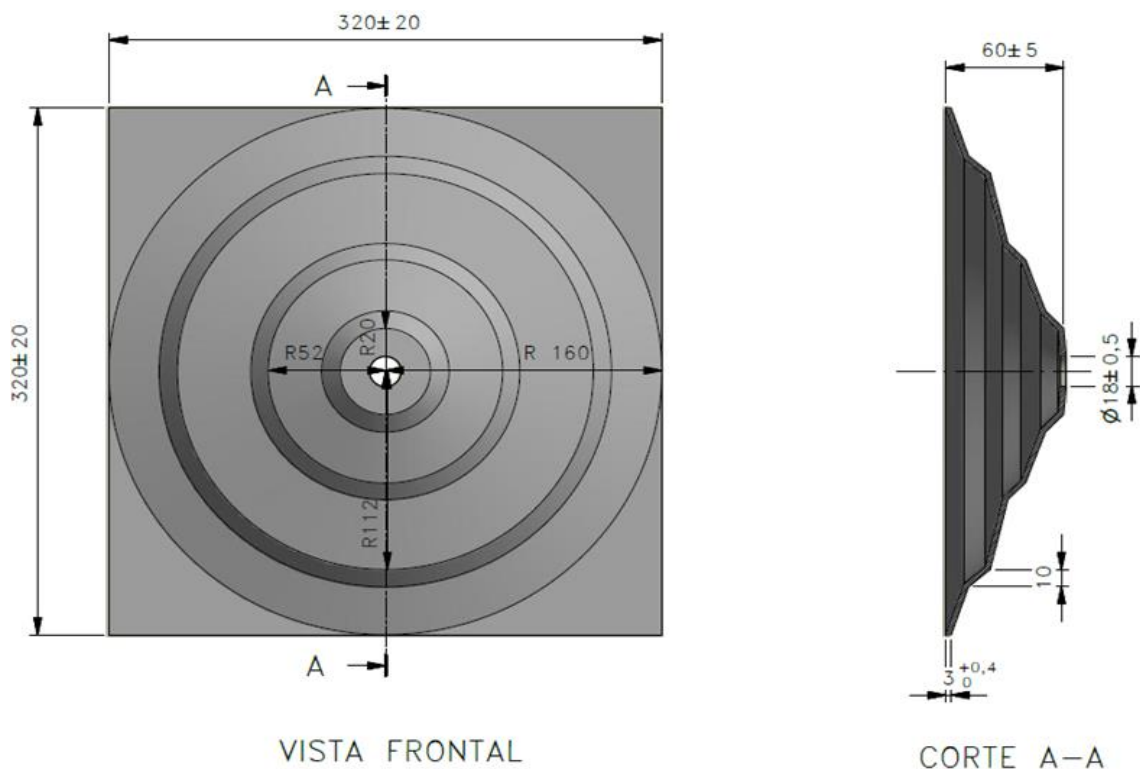
Figura 1 - Vistas da Chapa Para Âncora
